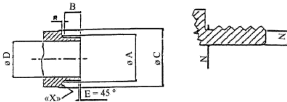
Рисунок 5 – Наружное цилиндрическое резьбовое соединение по ГОСТ 6357
