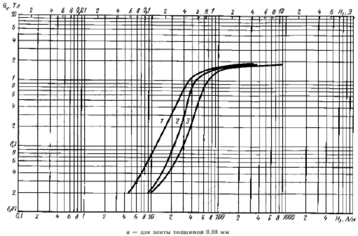
Кривые намагничивания стали марки 3424 (3360А) для частот: 1 — 400 Гц, 2 — 1000 Гц, 3 — 3000 Гц
