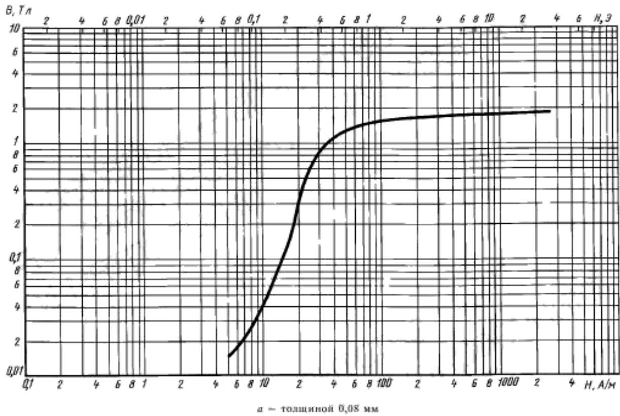
Кривые намагничивания стали марки 3424 (Э360А)
