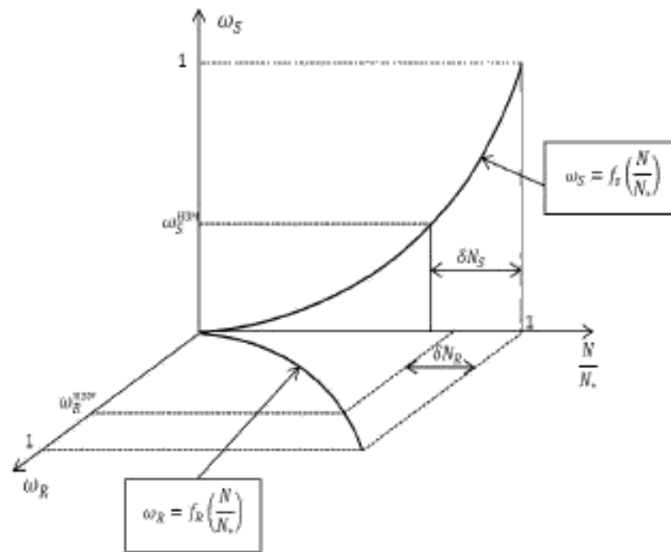
Рисунок 4 — Определение относительного остаточного ресурса
