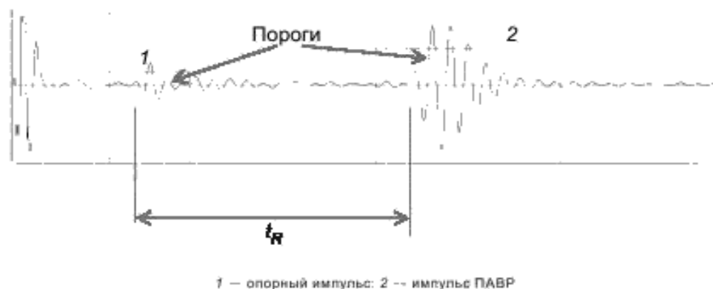
Рисунок 2 — Типичная осциллограмма при измерении преобразователем ПАВР
