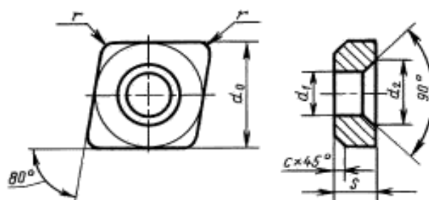
Размеры, мм
