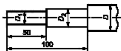
Рисунок А.1 — Форма образца
